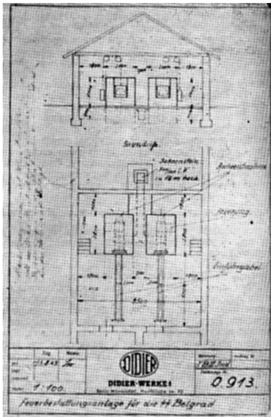
Plan krematorija za logore na Banjici i Sajmištu
